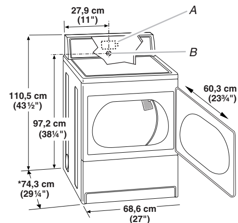
A. Tapa del bloque de terminal B. Protector del cable de suministro eléctrico
