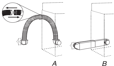
A. Allacciamento consigliato (disponibile solo con sezione a gomito) B. Allacciamento a periscopio
