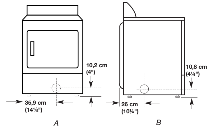
A. Evacuation à l'arrière B. Evacuation du côté gauche ou droit
