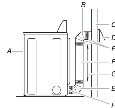
F. Conduit métallique rigide ou souple
